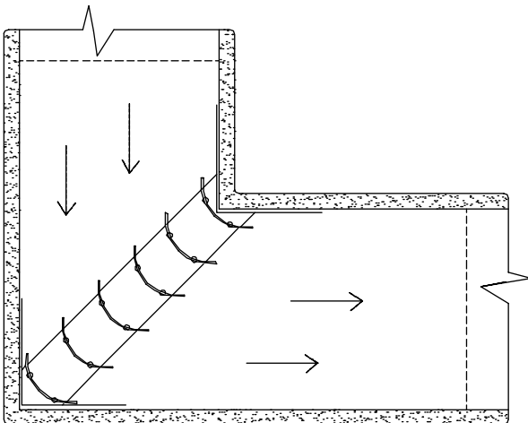
Cotovelo com lados iguais.
