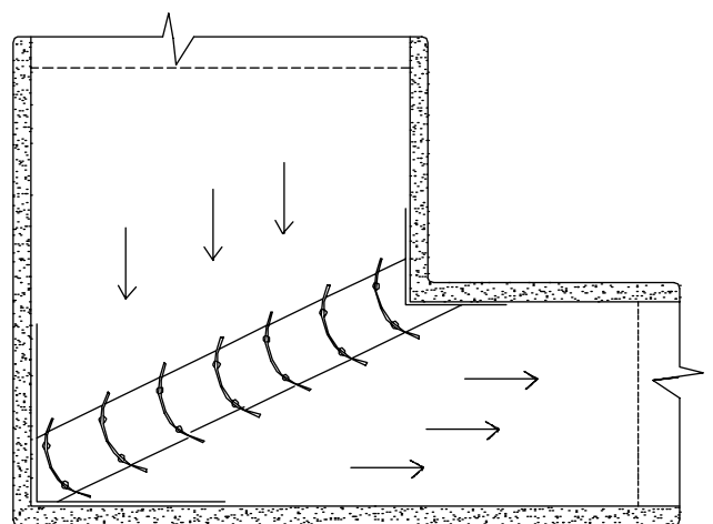
Cotovelo com lados desiguais.
