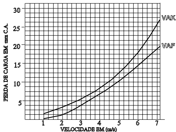
GRÁFICO DE PERDA DE CARGA
