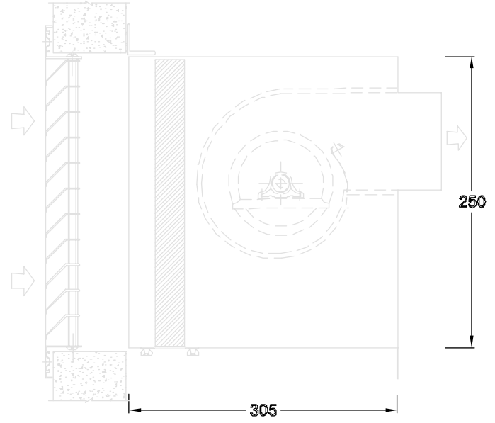
VISTA LATERAL
