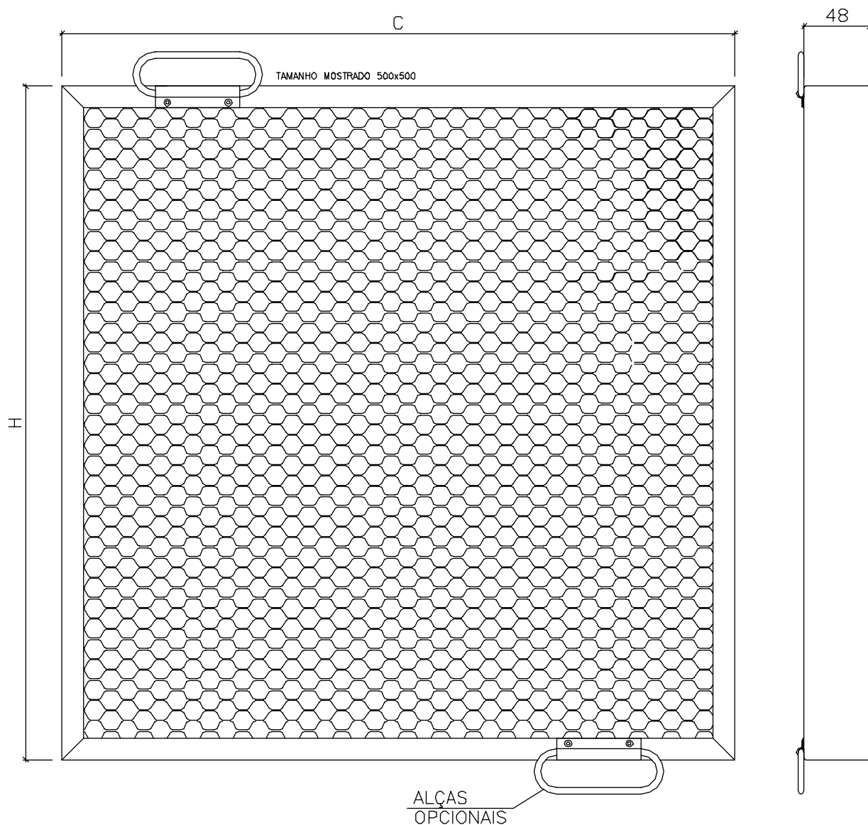
TAMANHOS NOMINAIS FABRICADOS (mm) DIMENSÕES EFETIVAS -5 mm
