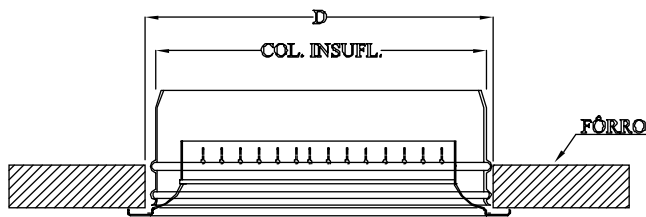
DETALHE : MONTAGEM EM FÔRROS
