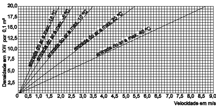
GRÁFICO DE DENSIDADE DE KW x VELOCIDADE DO AR
