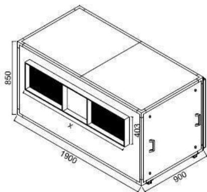
CFB 20 D 13.600 m 3 /h x 25 mmca 15 /15 duplex ventilador: 15 /15 duplex Otam motor: 4,0hp peso: 170Kg
