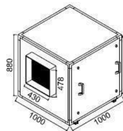
CFB 12,5 S 8500 m 3 /h x 20 mmca ventilador: 18/13 otam motor: 3hp peso: 110Kg
