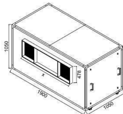
CFB 25D 17.000 m 3 /h x 25 mmca 18 /13 duplex ventilador: 18 /13 duplex Otam motor: 5,0hp peso: 180Kg
