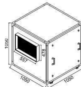
CFB 15 S 10.200 m 3 /h x 20 mmca ventilador: 18/18 otam motor: 3hp peso: 120Kg
