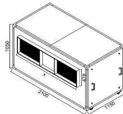
CFB 30D 20.400 m 3 /h x 25 mmca 18 /18 duplex ventilador: 18 /18 duplex Otam motor: 7,5hp peso: 190Kg
