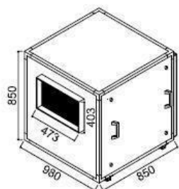
CFB 10S 6800 m 3 /h x 20 mmca ventilador: 15/15 otam motor: 2hp peso: 85Kg
