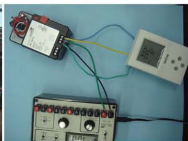
Teste de servomotores proporcionais
